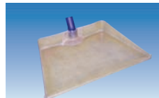
Art.-Nr. 2230009800 Schwimm-Saugschaufel zum Absaugen von Öl auf kleinen Wasserflächen
